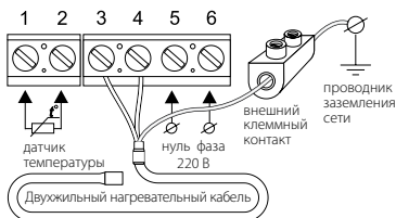
Схема подключения нагревательного кабеля «РУССКОЕ ТЕПЛО» РТ
